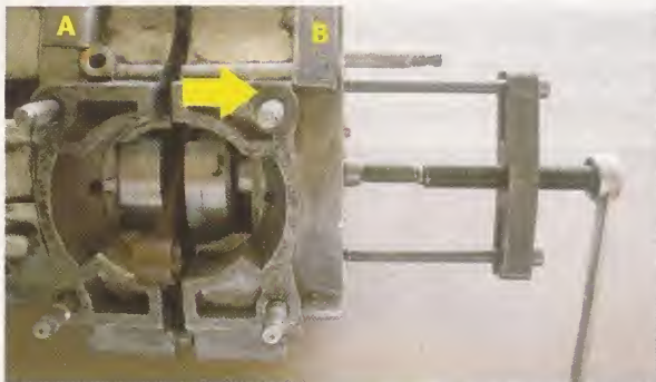
Acción de separado de carcasas
